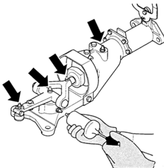
شکل ۲۷: ترانسمیشن خشک و نقاط گریس خور آن
