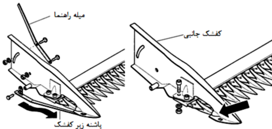
شکل ۶: مونتاژ کاتربار ۱۱۵ سانتی متری
