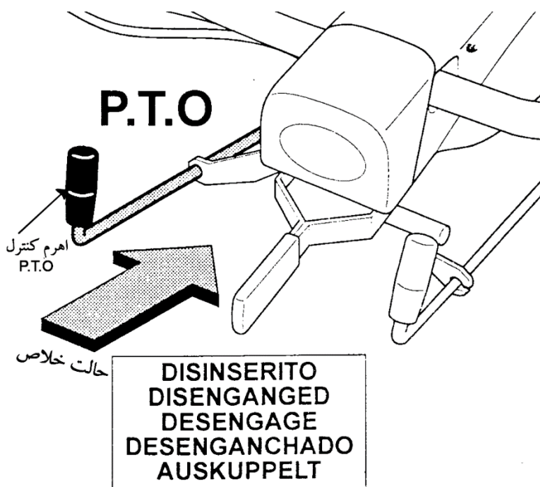
شکل ۱۷: محل قرار گیری اهرم کنترل PTO
