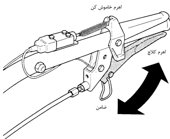
شکل ۱۴: اهرم کلاچ، اهرم خاموش کن و ضامن
