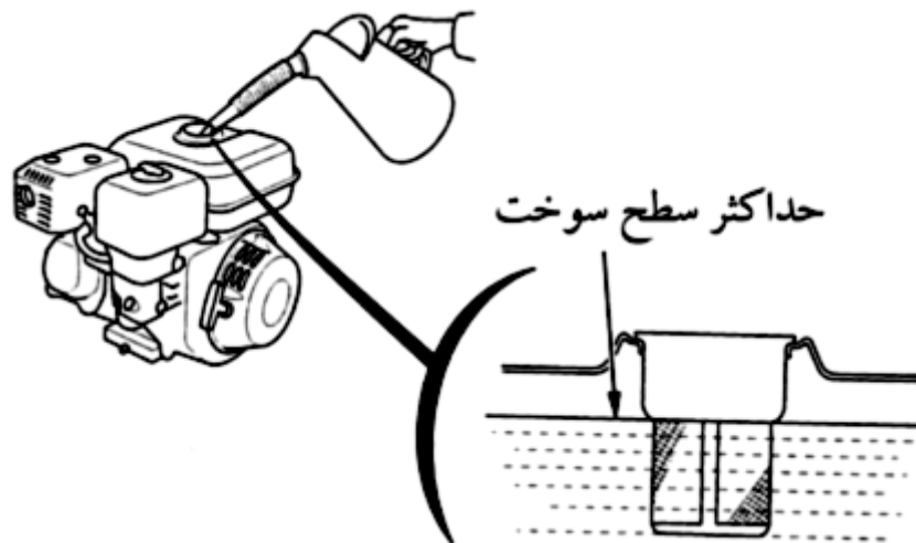
شکل ۸: سوختگیری موتور
