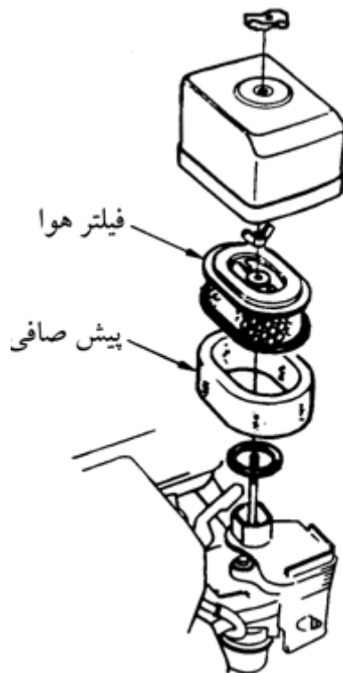
شکل ۲۰: محل قرار گیری فیلتر هوا و پیش صافی
