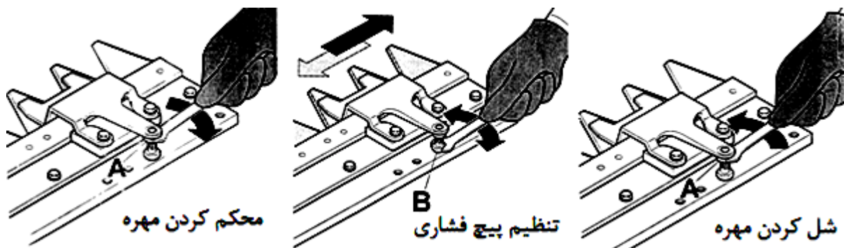
شکل ۳۳: مراحل تنظیم تیغه در کاتر بار ۱۰۰ سانتی متری
