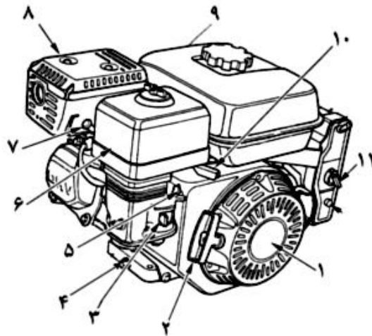
شکل ۱: اجزای موتور
