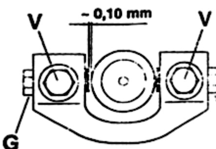
شکل ۳۲: تنظیم خلاصی کوپلینگ حرکت تیغه
